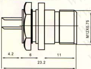
X12型 KnL型插座 X12 TYPE KnL TYPE SOCKET
