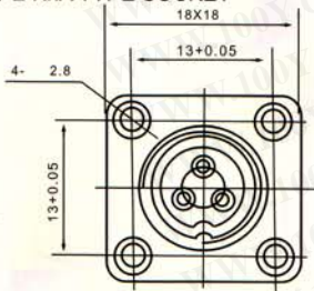
X12型 KnA型插座 X12 TYPE KnA TYPE SOCKET
