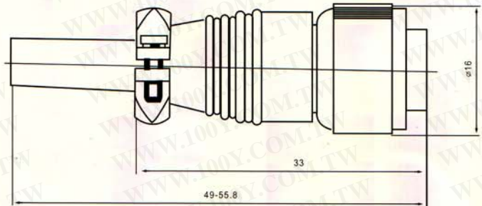
X12型 KnP型插座 X12 TYPE KnP TYPE SOCKET
