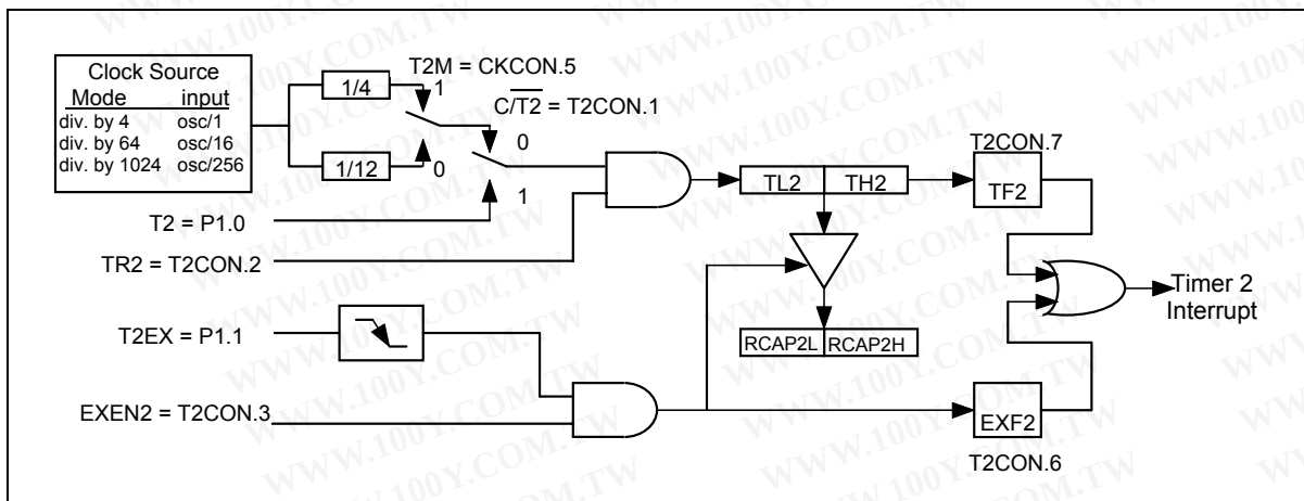
图14: 16位捕捉模式
