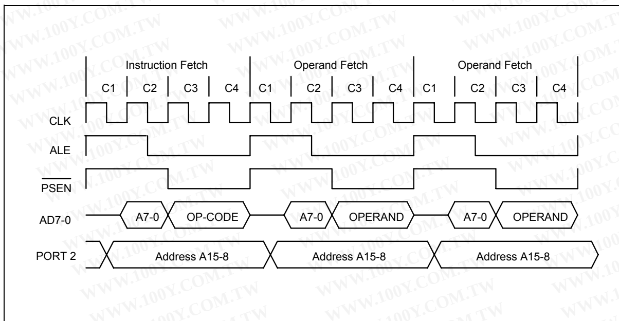
图5：3周期指令时序
