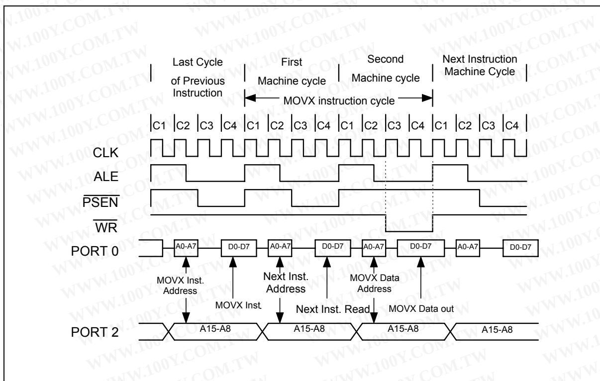
图8: STRETCH=0时的外部数据存储器访问时序
