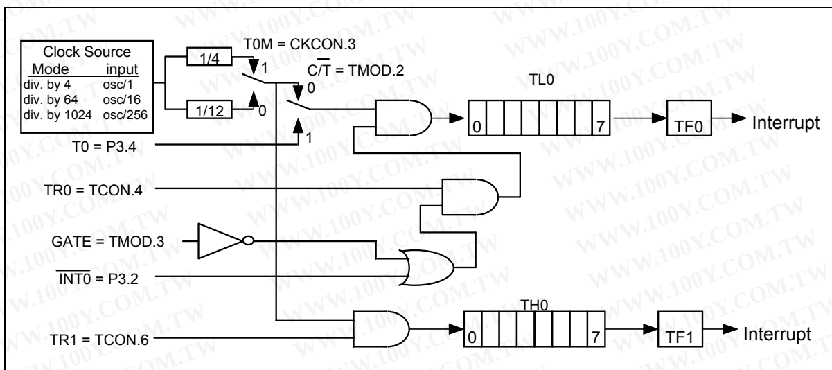
图3: 模式0下的定时器0
