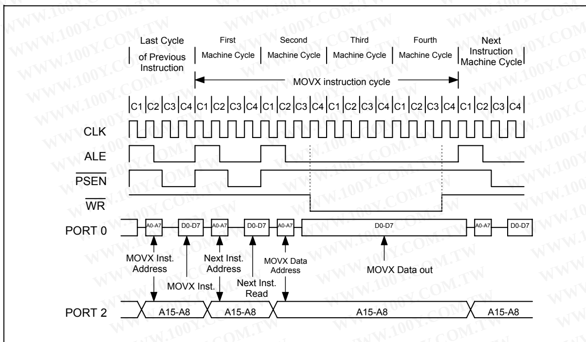
图10: STRETCH=2时的外部数据存储器访问时序
