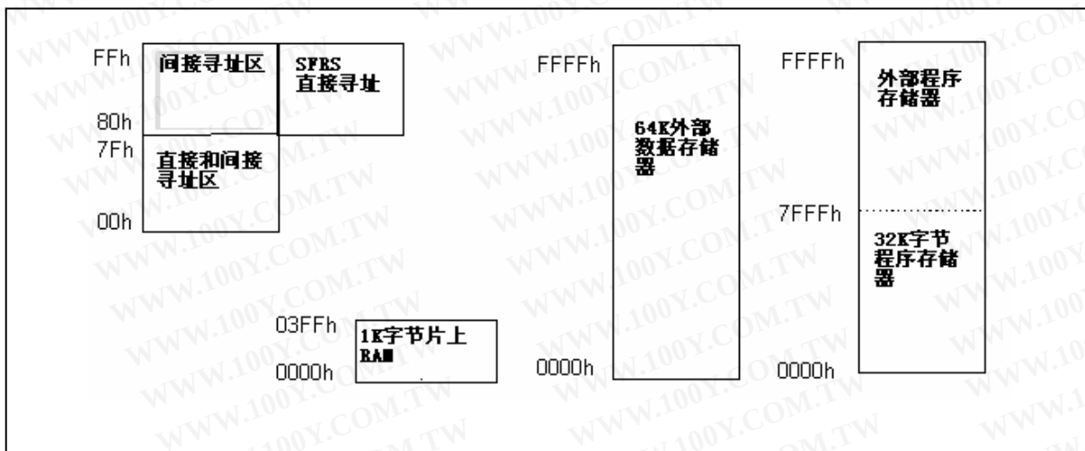
图1:存储器映射
