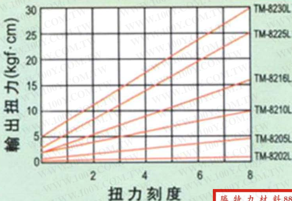
輸出扭力曲綫表
