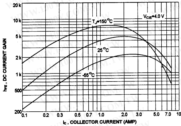
NPN TIP120,TIP121,TIP122
