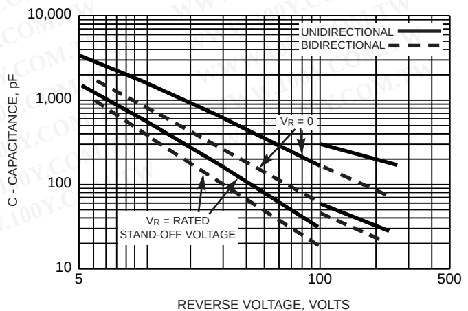
FIG. 6 - CAPACITANCE
