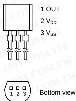
(1) TO-92
