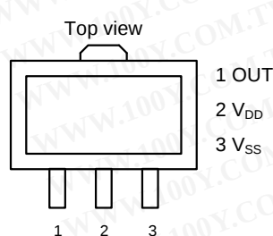
(2) SOT-89-3
