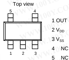
(3) SOT-23-5
