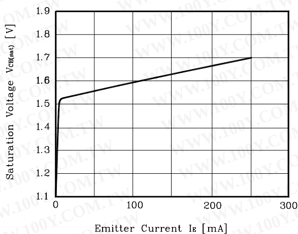
Fig. 2 V_{CE} - I_E
