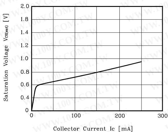
Fig. 1 V_{CE(sat)} - I_C
