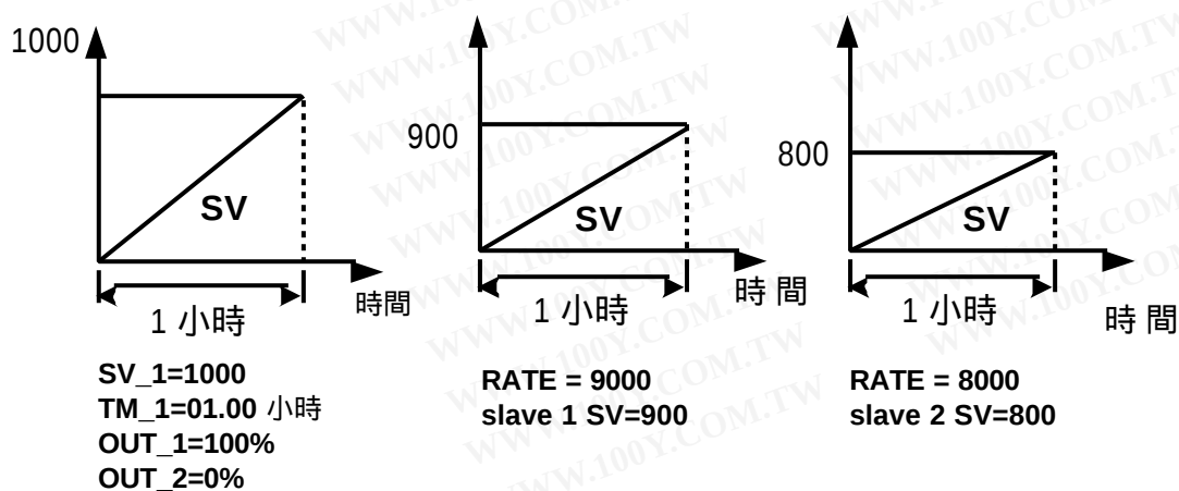
時序圖
