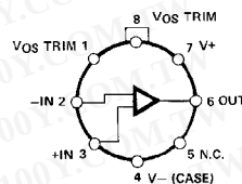
TO-99 (J-Suffix)
