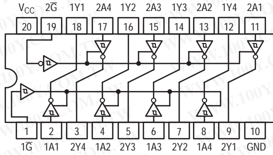
SN74LS240
