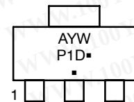
SOT-223 CASE 318E-04 STYLE 1
