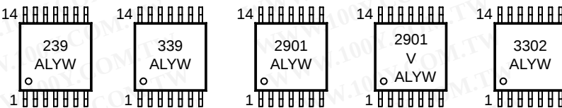
TSSOP-14 DTB SUFFIX CASE 948G
