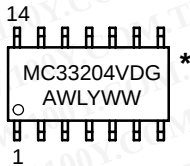
SO-14 VD SUFFIX CASE 751A
