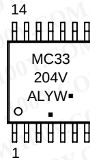
TSSOP-14 DTB SUFFIX CASE 948G
