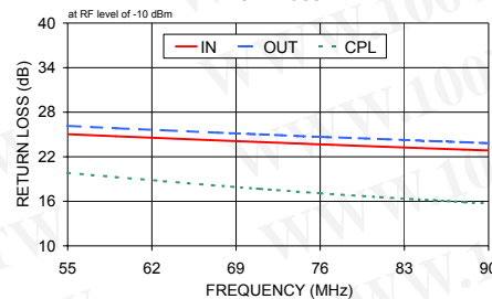
ZDC-20-3-75-1 RETURN LOSS
