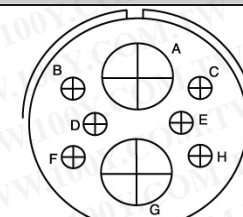
32-15 6-#12,2-#0 D
