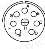
20-9 7-#16,1-#12 BAL=A
