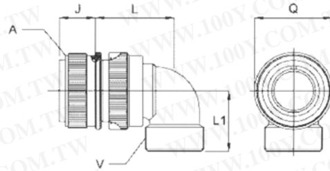
DIMENSIONS IN INCHES 英呎規格
