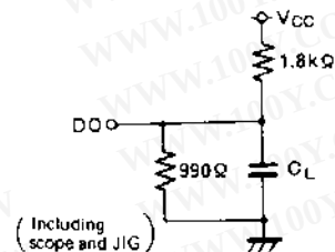
Fig. 1 Output load
