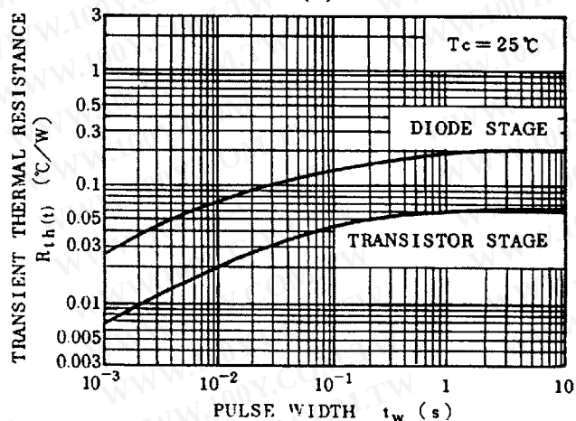
R_{th}(t) - t_w
