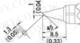
T10-BC4 Shape-4BC Bevel T10-BCF4 ※
