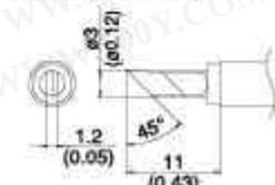
T12-KU SHAPE-KU
