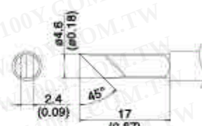
T12-KU SHAPE-KU
