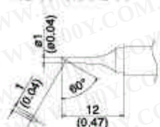
T12-C1 SHAPE-1C
