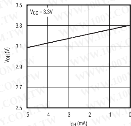
DQ OUTPUT-VOLTAGE HIGH vs. DQ OUTPUT-CURRENT HIGH
