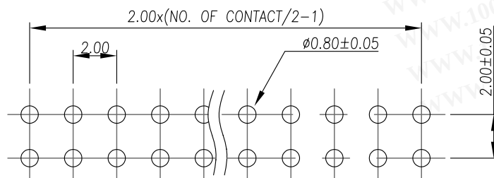
P.C.B. LAYOUT
