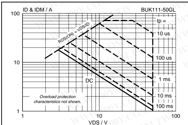
Fig.37. Safe operating area, V_{PS} = 0\text{ V} , T_{mb} = 25^\circ\text{C} . I_D & I_{DM} = f(V_{DS}) ; I_{DM} single pulse; parameter t_p
