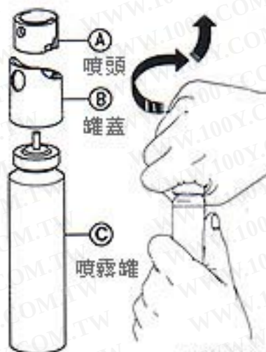
分解／組合示意圖
