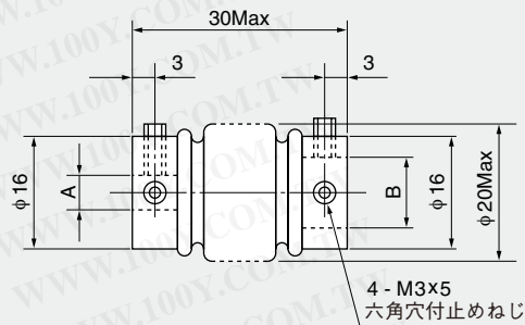
Dimension mm 寸法 mm
