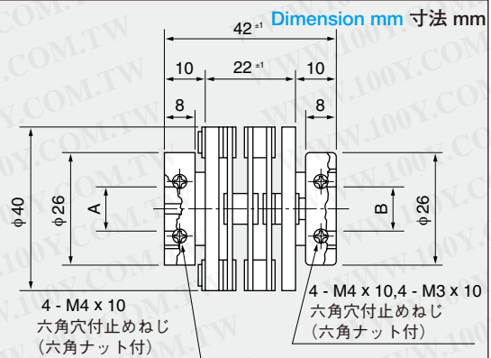
Dimension mm 寸法 mm
