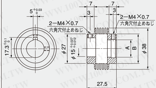
Dimension mm 寸法 mm
