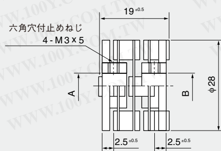
Dimension mm 寸法 mm
