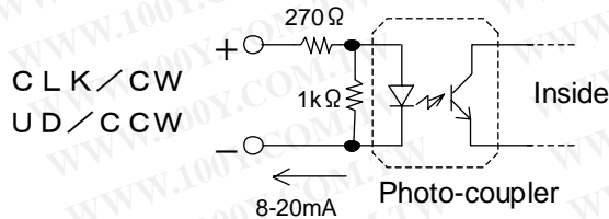
Fig.10. Clock Inputs
