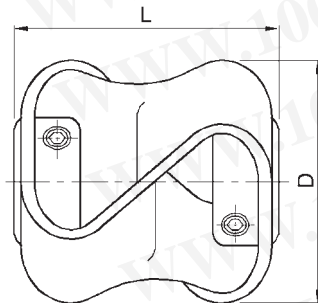
Coupling Type 047
