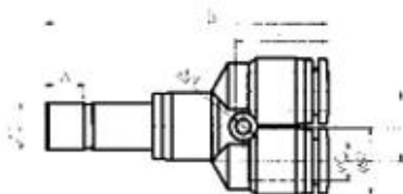
● YPWJ/TPWJ Y型减径三通
