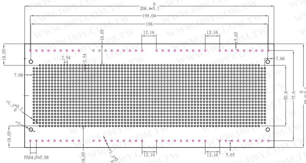
D12MG-PCB-A
