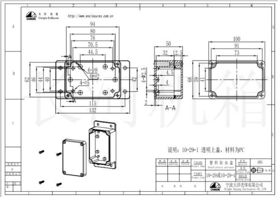
产品结构图
