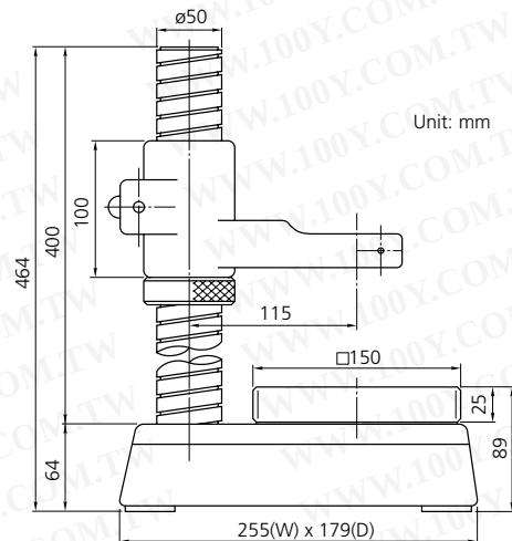
215-504 (ø8mm) 215-505 (ø20mm)
