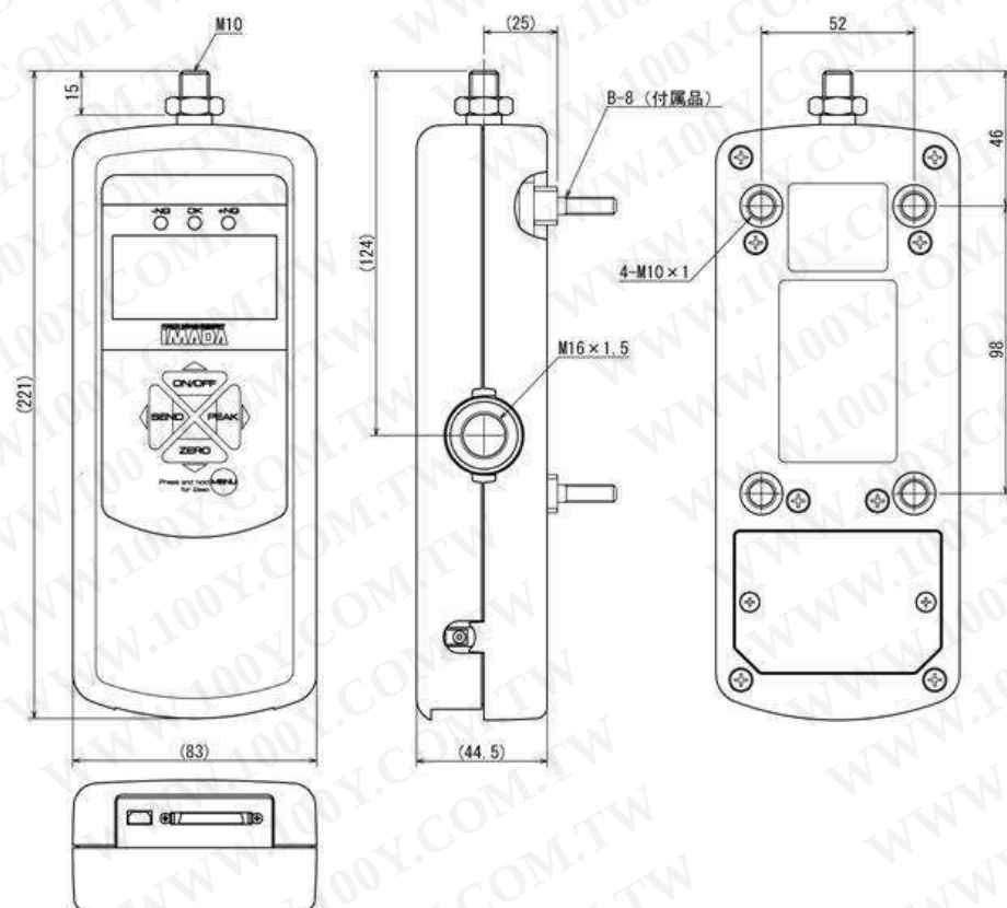
[外観図：2500N～5000N]
