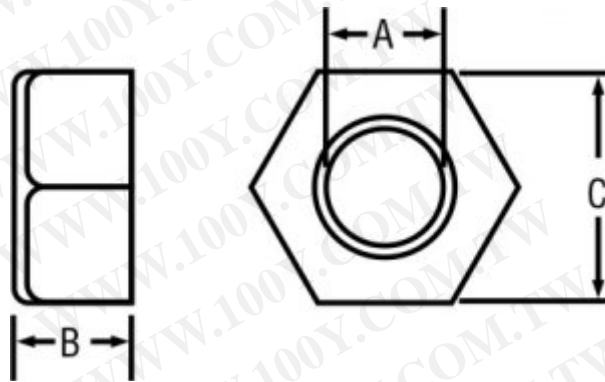
公制塑膠螺母工程圖
