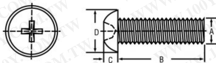
十字圓柱頭塑膠螺絲緊固件工程圖
