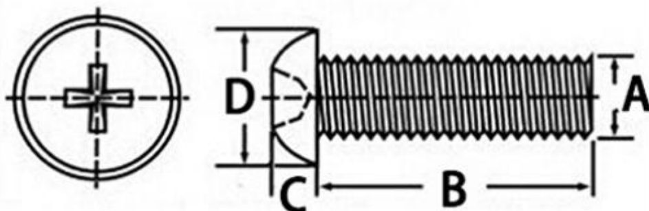
测量示意图
