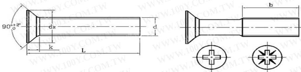
测量示意图
