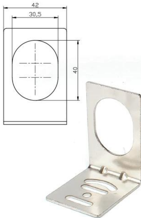
M30 L形弯角支架
