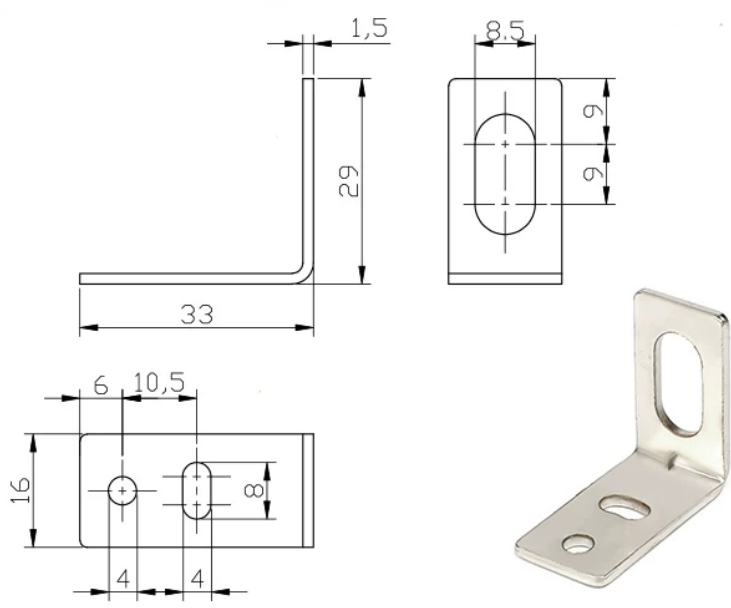
M8 L形弯角支架
