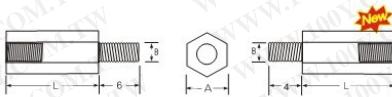
內外螺紋六角隔離柱工程圖
