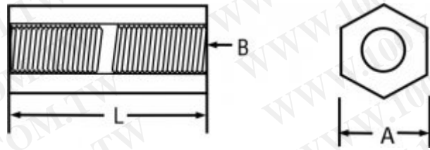
內螺紋六角隔離柱工程圖
