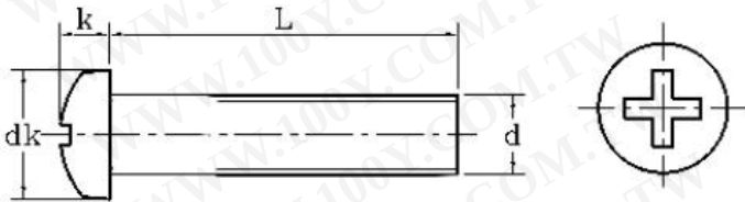
图纸示意图
