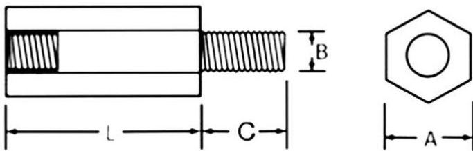
測量示意图
