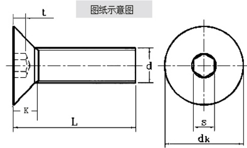
图纸示意图
