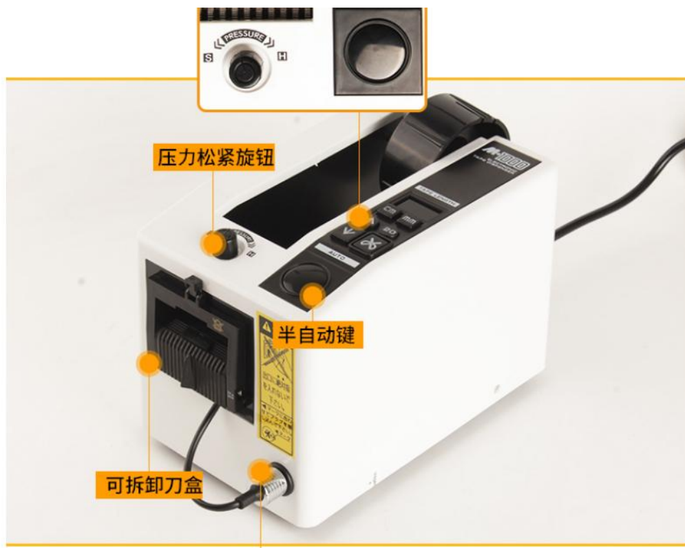
胶纸座
