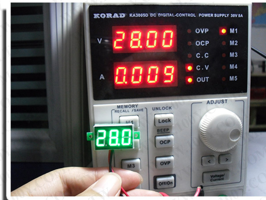
BV102与可调稳压电源电压对比图
