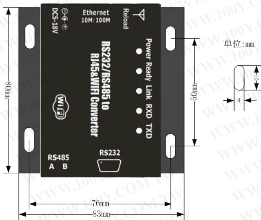
图 5 602/604/610 外观尺寸图
