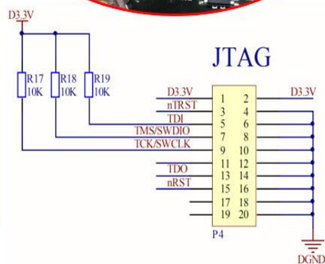
JTAG仿真接口电路
