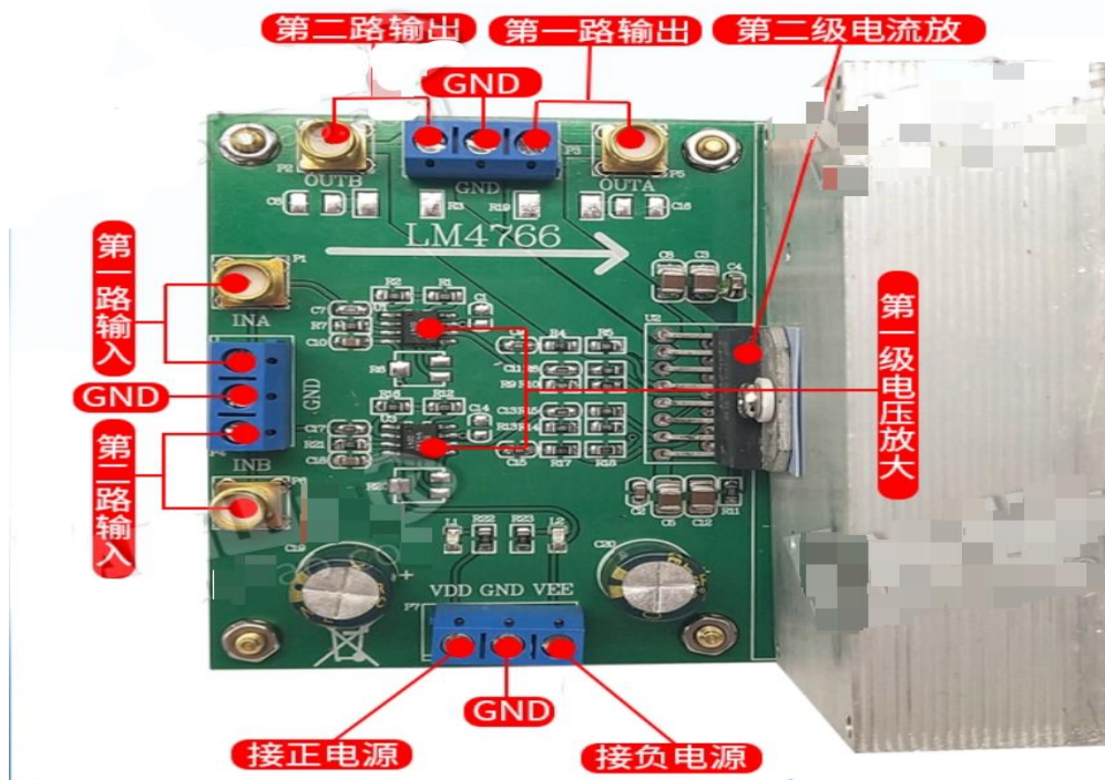
模块接口图
