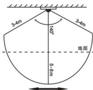
天花板安装图示
