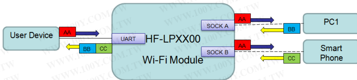
Figure 13. 双 Socket 数据流向示意图
