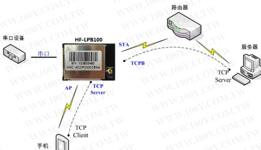
Figure 10. HF-LPB100 的 AP+STA 组网结构
