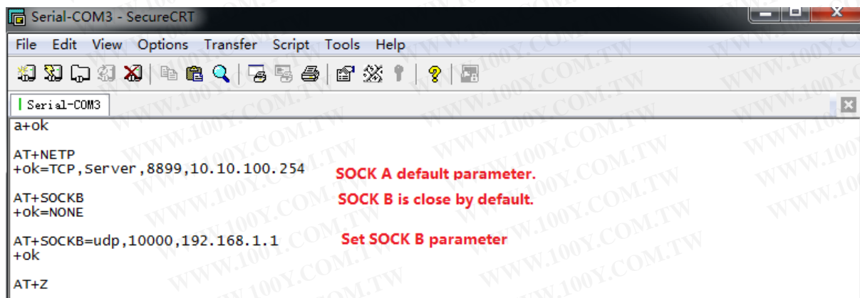
Figure 12. 双 Socket 设置命令
