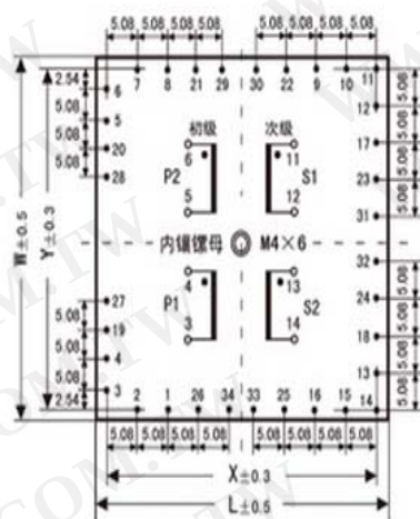
底视图
