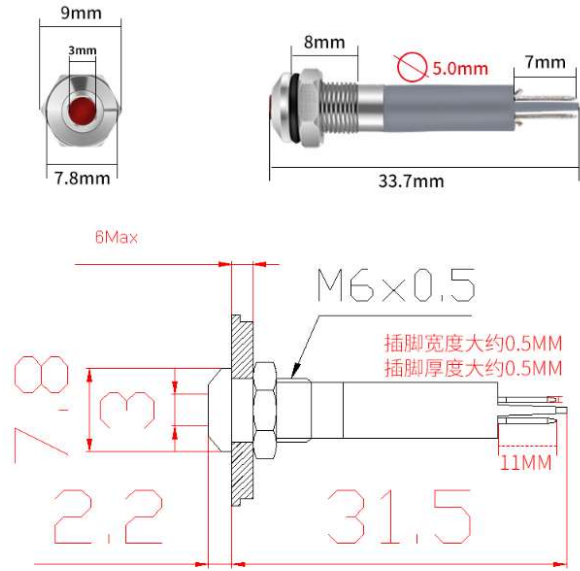
开孔6MM平头款
