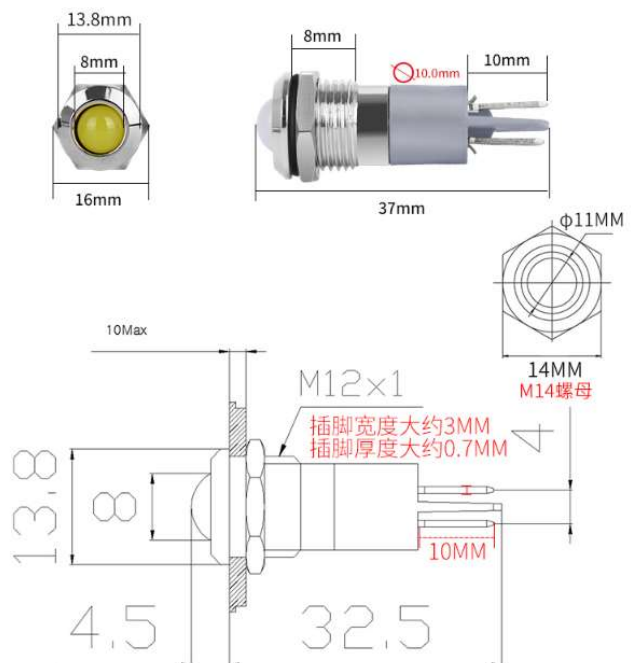
开孔12MM高头款
