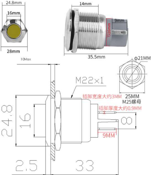
开孔22MM平头款
