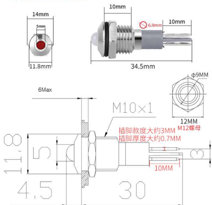
开孔10MM高头款
