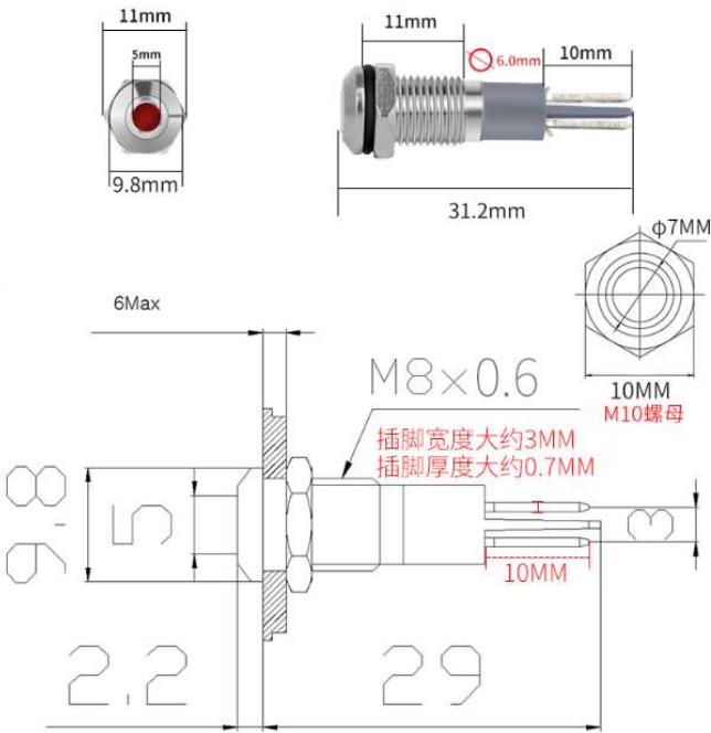
开孔8MM平头款
