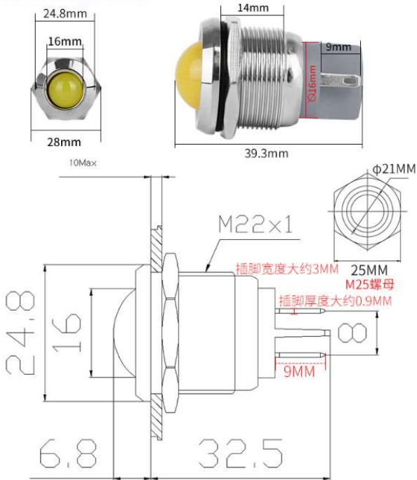
开孔22MM高头款
