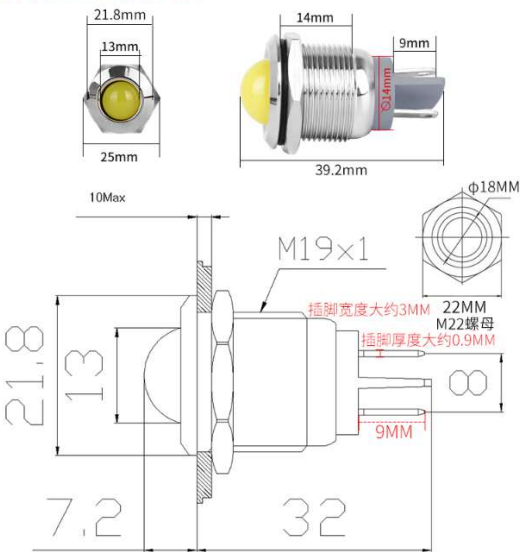
开孔19MM高头款
